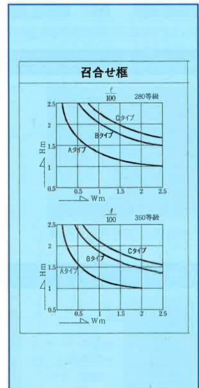
〈製作限界〉
